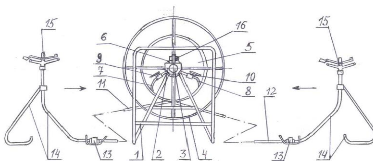
Рисунок 4 - Передвижная малоинтенсивная дождевальная установка ПДУ – 33 1 – рама; 2 – опора рамы; 3 – полый вал; 4 – катушка; 5 – барабан; 6 – внутренняя труба; 7,8 – отвод; 9,10 – кран; 11,12 – полиэтиленовая труба \varnothing 32 , l = 50 м; 13 – муфта; 14 – опора; 15 – дождевальный аппарат; 16 – стопор
