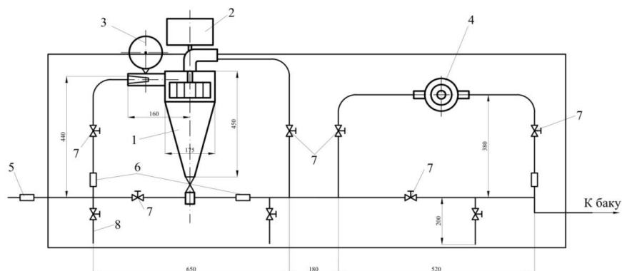
1-гидроциклон с гидротурбиной; 2-генератор; 3-дозатор для подачи песка; 4-гидротурбина с генератором-2; 5-электронный расходомер; 6- электронные датчики давления; 7- задвижки; 8- водослив; 9- насадок
