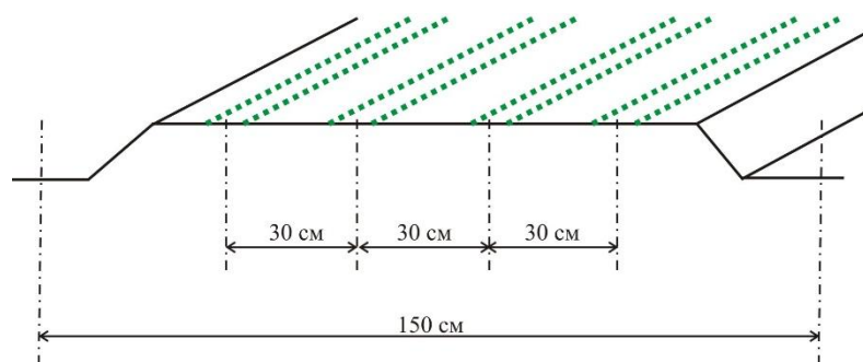
Рисунок 1 - 4-х рядная сдвоенная схема посадки лука
