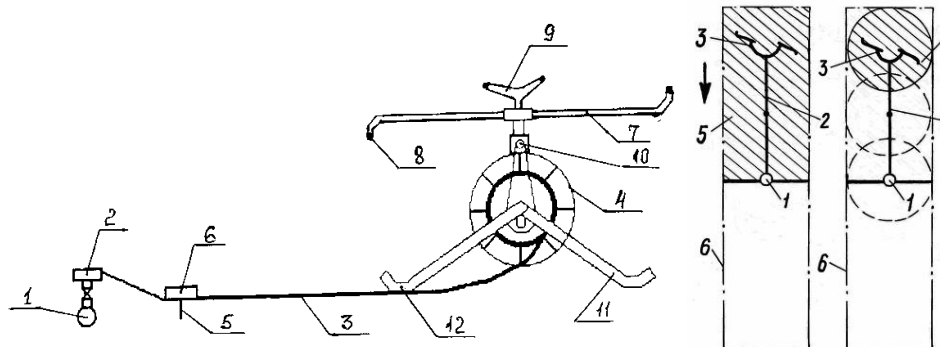
Рисунок 5 - Технологическая схема полива дождевальной установкой «ДШ-1» для орошения в теплицах рассады, выращиваемой в кассетах
