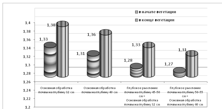
Рисунок – Влияние приемов различной обработки на объемную массу почвы в слое 0-30 см, г/см³
